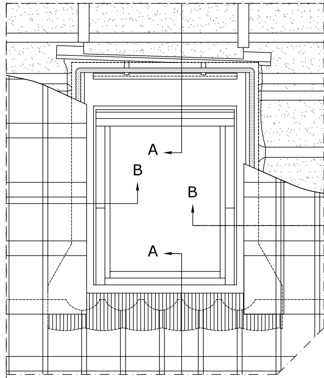
prerez A-A 1:5
